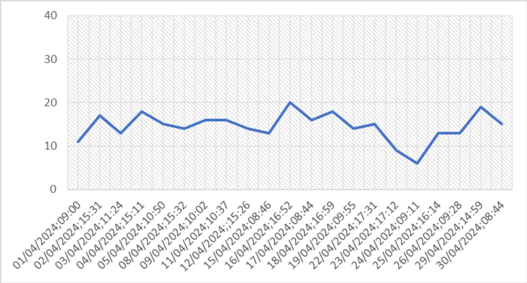
Gráfico 04 – Monitoramento de Pressão do PCP 03.
