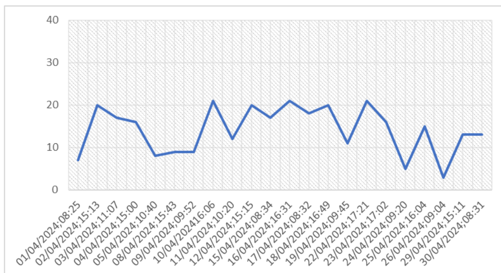
Gráfico 02 – Monitoramento de Pressão do PCP 01.
