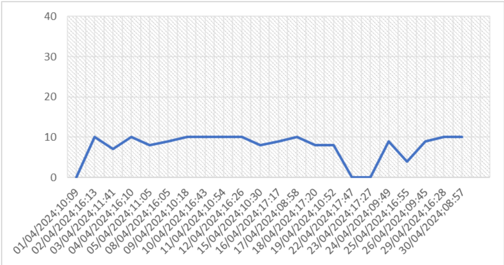
Gráfico 07 – Monitoramento de Pressão do PCP 06.
