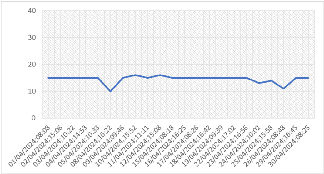
Gráfico 09 – Monitoramento de Pressão do PCP 08.
