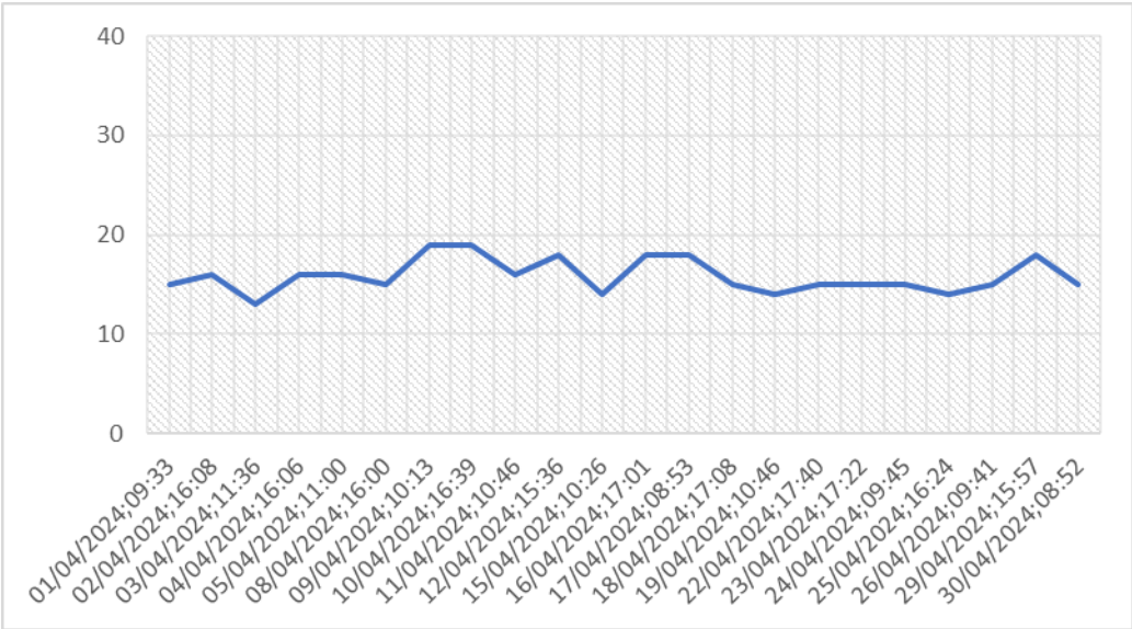
Gráfico 06 – Monitoramento de Pressão do PCP 05.
