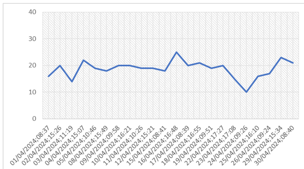
Gráfico 03 – Monitoramento de Pressão do PCP 02.
