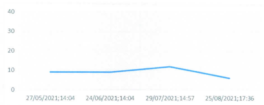
Gráfico 08 – Monitoramento de Pressão do PCP 07.
