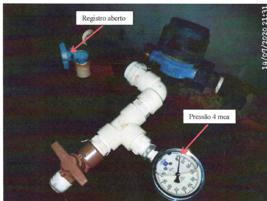
Imagem 06: Pressão 04 mca - Av. São Cristóvão, 2664, Recanto dos Pássaros II - HD Y16S441205.
