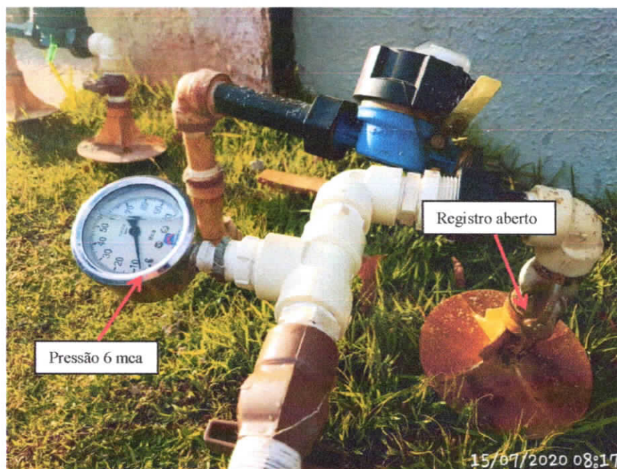
Imagem 05: Pressão 06 mca - Rua Ponta Grossa, 630, Cidade Alta - HD Y17T061911.
