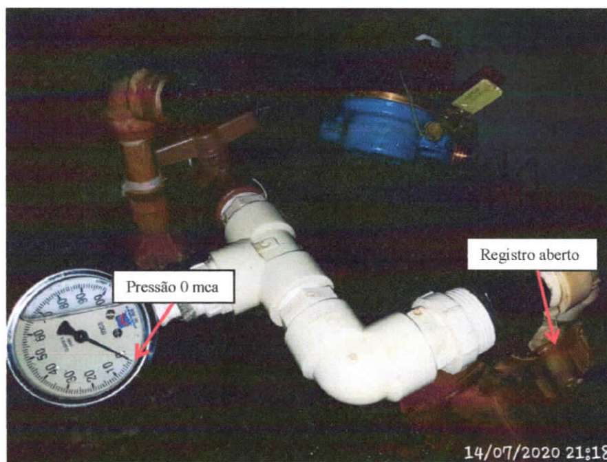
Imagem 04: Pressão 0 mca - Rua Ponta Grossa, 630, Cidade Alta - HD Y17T061911.
