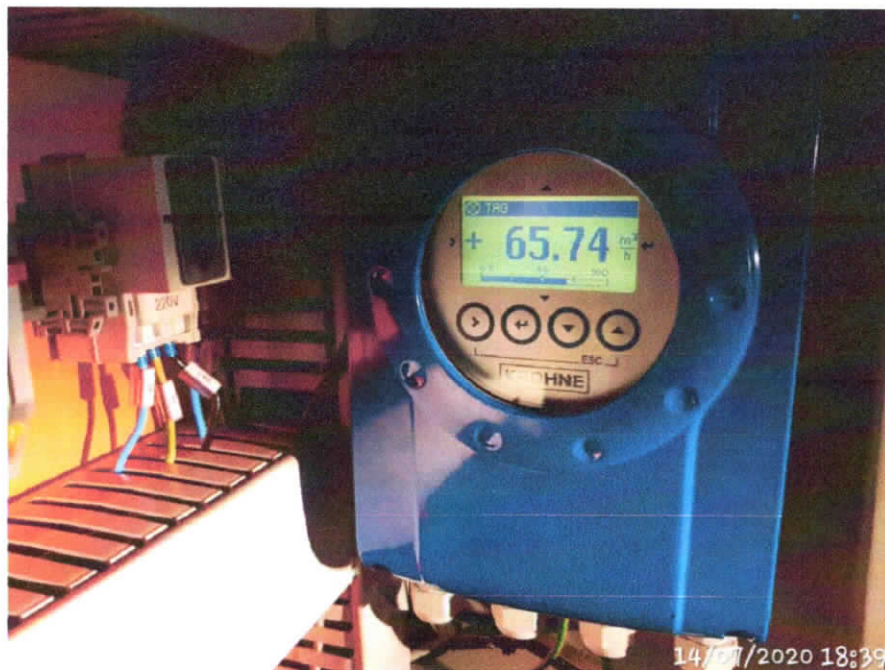
Imagem 02: Detalhe da vazão instantânea em m³/h do poço 13.
