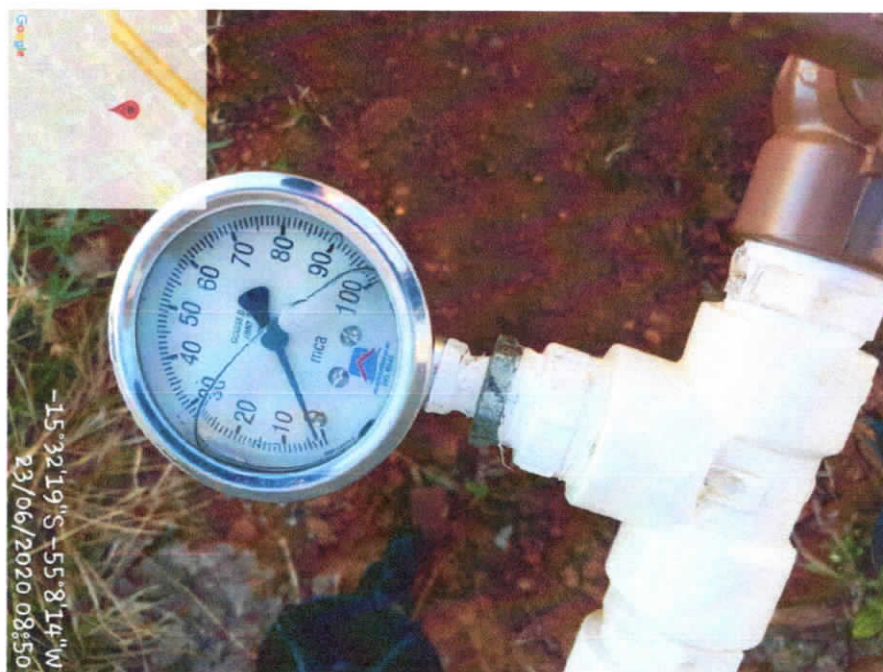
Imagem 01: Medição de pressão na Rua Francisco Beltrão, 743, Cidade Alta – HD: Y16S441205.
